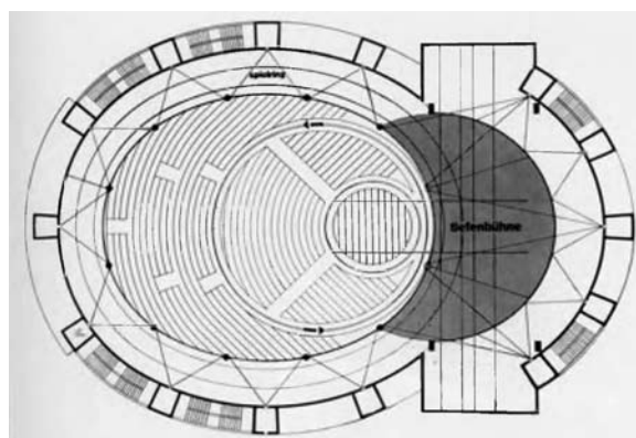
Nacrti za totalni teatar, 1927. iz: Siegfried Giedion, Walter Gropius. Mensch und Werk , Verlag Gerd Hatje Stuttgart, 1954, str. 151, 154, 155, 156, 157.
